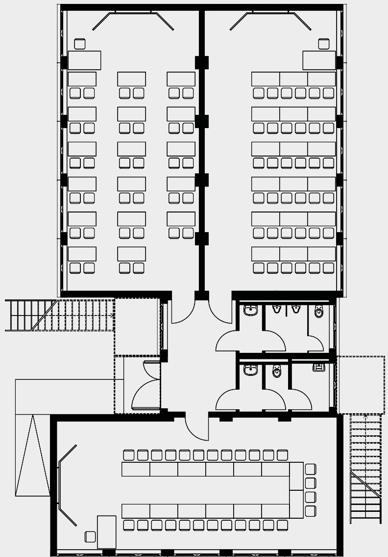
Grundrissbeispiel: Schule
