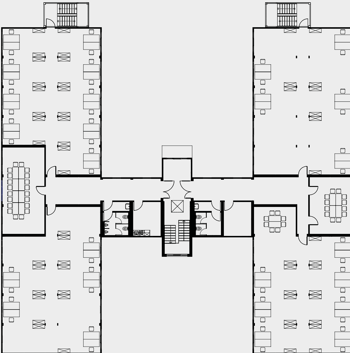
Grundrissbeispiel: Großraumbüro
