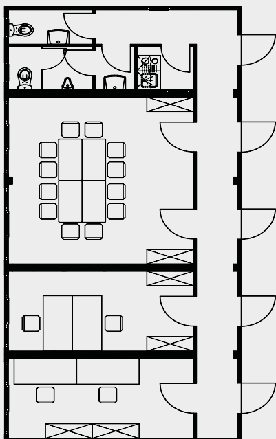
Grundrissbeispiel: Baustellenbüro
